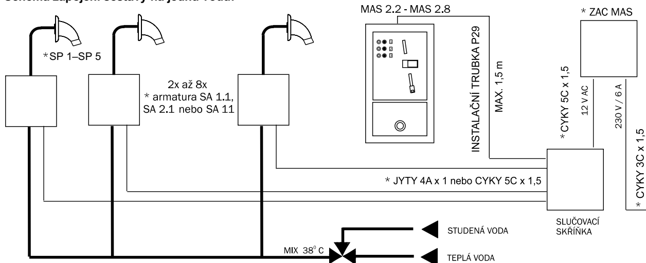
Schéma zapojení sestavy na jednu vodu:
