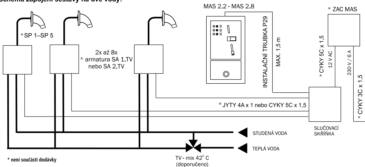
Schéma zapojení sestavy na dvě vody:
