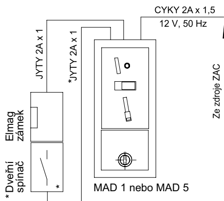
Schéma zapojení kompletní sestavy
