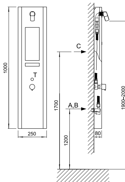
A - STUDENÁ VODA trubka G1/2" vnitřní B - TEPLÁ VODA trubka G1/2" vnitřní C - EL. PŘÍVOD kabel CYKY 2A x 1,5 T - OVLÁDACÍ TLACÍTKO (u AUS 3P)
