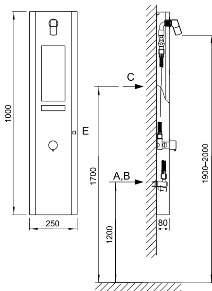
A - STUDENÁ VODA trubka G1/2" vnitřní B - TEPLÁ VODA trubka G1/2" vnitřní C - EL. PŘÍVOD kabel CYKY 2A x 1,5 E - ZÓNA SNÍMÁNÍ
