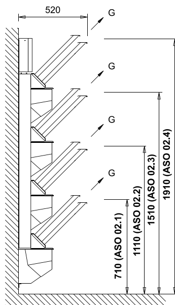
C - EL. PŘÍVOD G - VÝSTUP VZDUCHU
