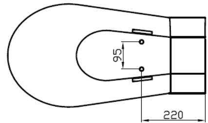
pohled zespodu - otvory pro svorníky M12
