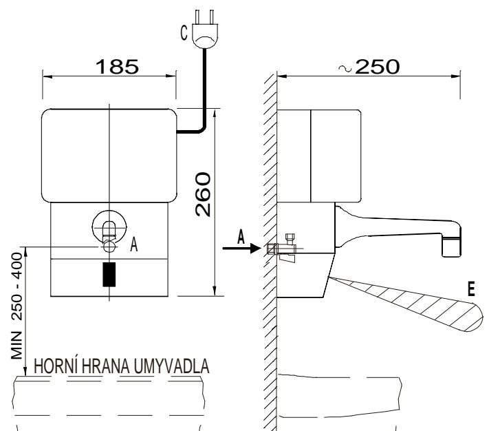
A - STUDENÁ VODA trubka G 1/2" C - EL. PŘÍVOD E - ZÓNA SNÍMÁNÍ
