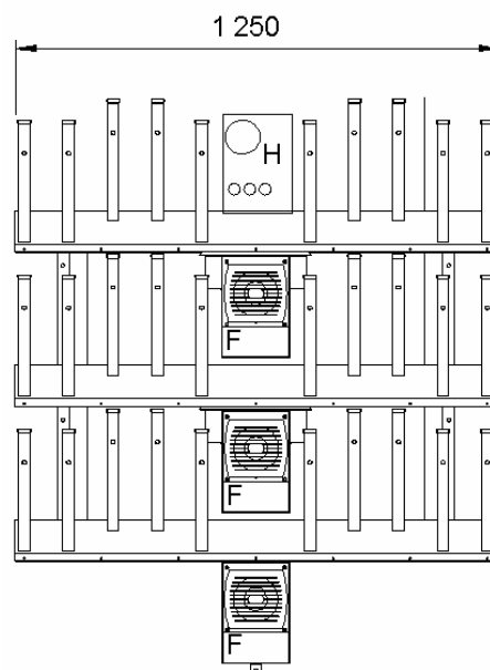
H - ovládací panel G - výstup vzduchu F - ventilátor
