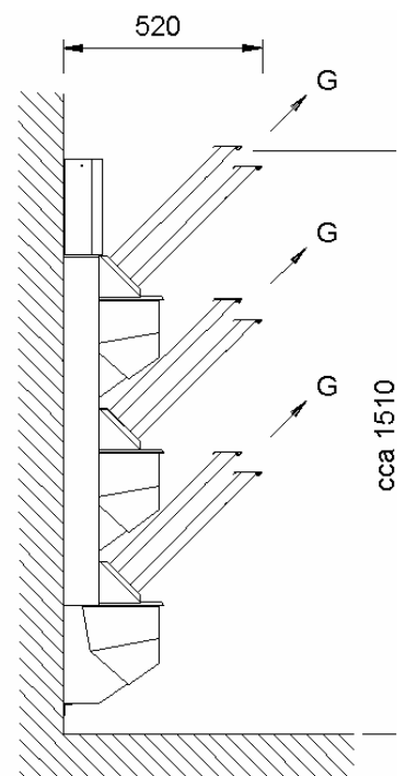
H - ovládací panel G - výstup vzduchu F - ventilátor
